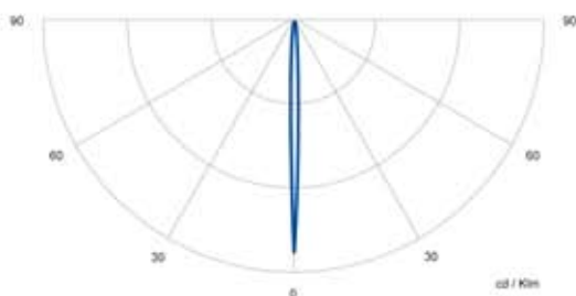
Curva Fotométrica
