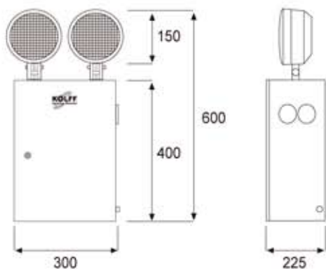
Dimensiones (mm)
