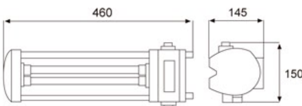
Dimensiones (mm)
