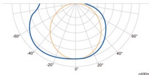
Curva Fotométrica
