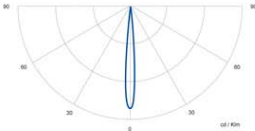
Curva Fotométrica
