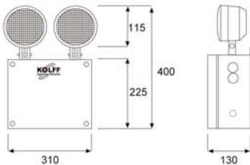
Dimensiones (mm)
