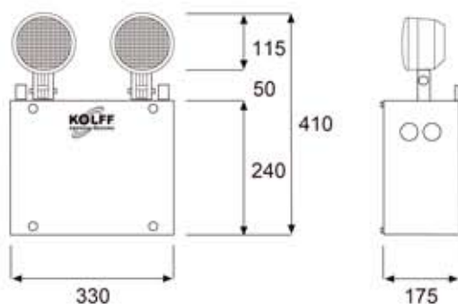
Dimensiones (mm)
