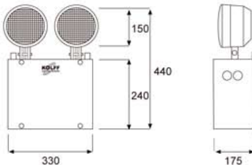
Dimensiones (mm)
