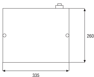
Dimensiones (mm)
