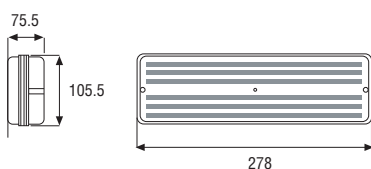
Montaje Superficial
