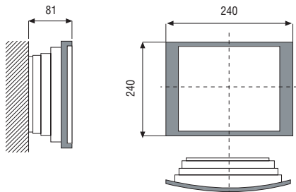
Dimensiones (mm)
