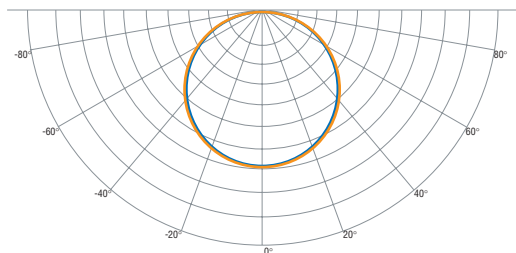
Curva Fotométrica
