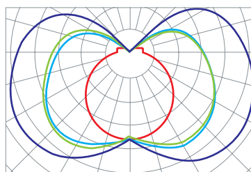
Curva Fotométrica
