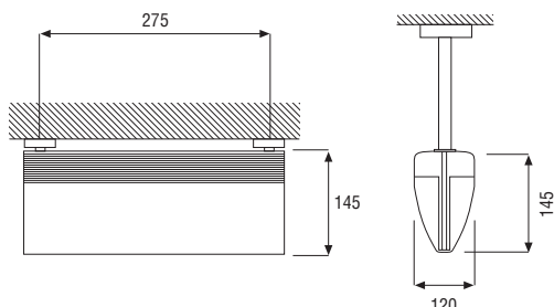
Dimensiones (mm)
