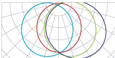
Curva Fotométrica
